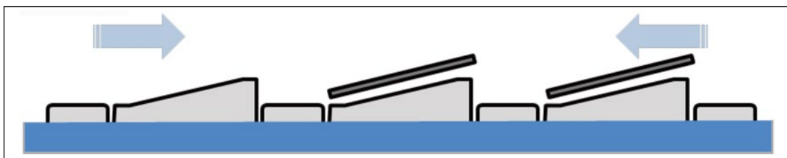
▲圖十九 系統組件各材料熱膨脹係數不同，長期造成浮台與模組間隙變大
