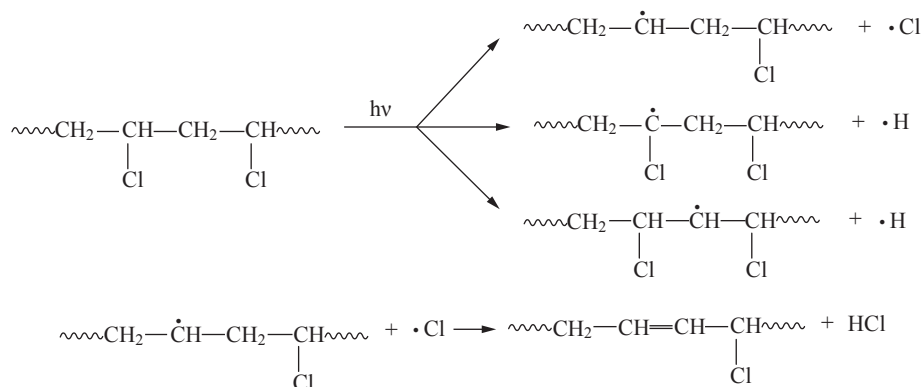
▲圖一 PVC光裂化機制 (2)
