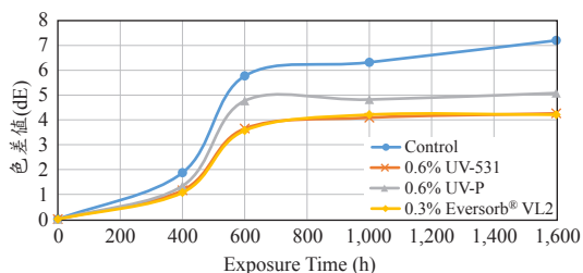
▲圖五 白色PVC添加不同類型的紫外光吸收劑，經耐候測試其色差值變化（彩圖請見材料世界網）
