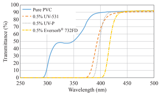
▲圖三 PVC添加不同紫外光吸收劑的紫外-可見光光譜圖(厚度1.6mm)(彩圖請見材料世界網)
