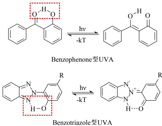
▲圖二 紫外光吸收劑作用機制 (3)
