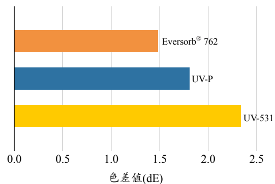
▲圖四 透明PVC添加0.5%不同類型的光安定劑(厚度3.2 mm)，照射1,000小時色差值變化
