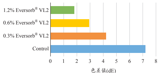
▲圖六 經過耐候測試1,600小時，白色PVC添加不同濃度Eversorb® VL2的耐候表現
