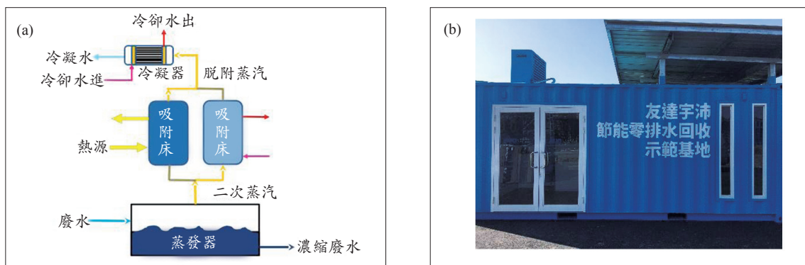
▲ 圖一 (a)友達宇沛「常溫蒸發零排技術」原理；(b)友達宇沛「節能零排水回收」示範基地
