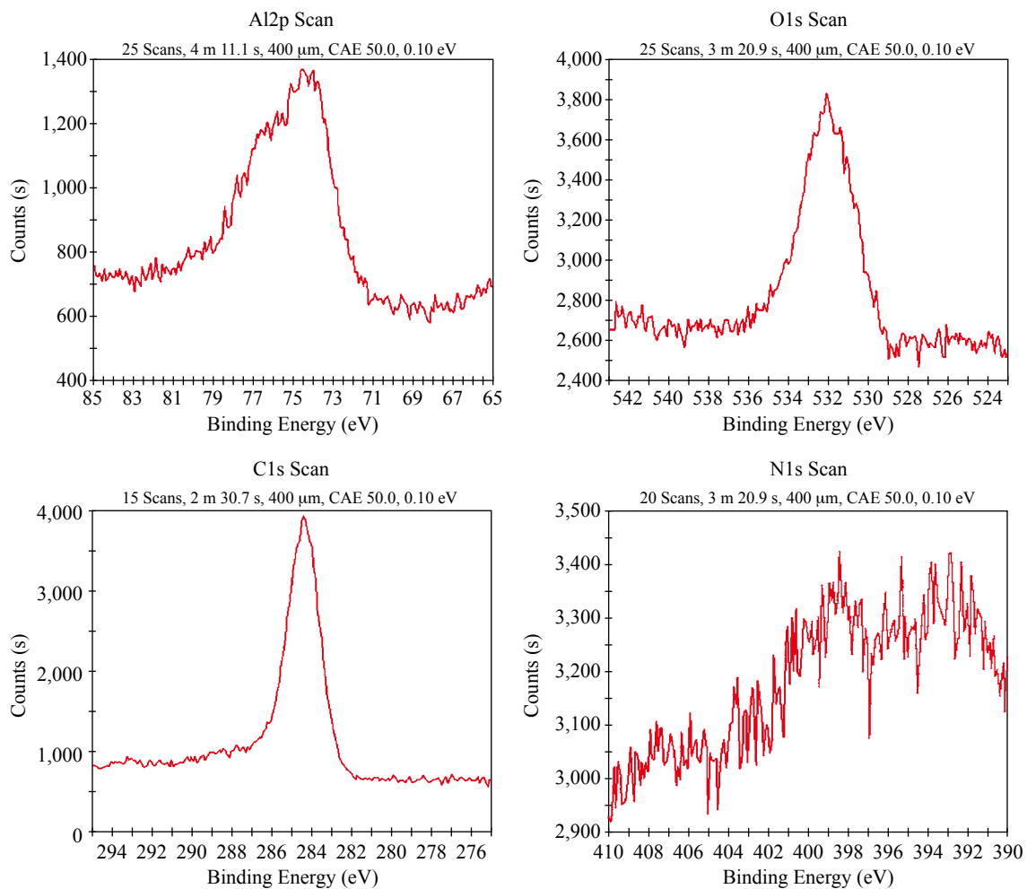
▲圖三 製備AlN膜的XPS分析結果
