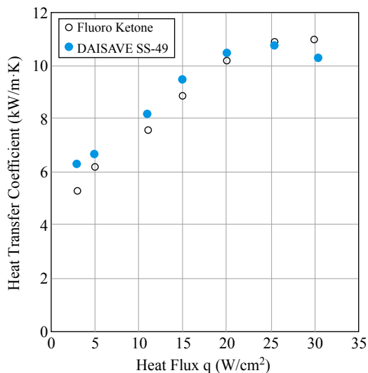
▲圖二 沸騰傳熱率的測試結果
