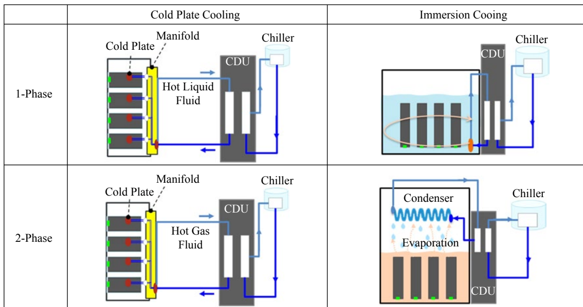
▲圖一 Data Center伺服器業界目前市場主流之冷卻方式（彩圖請見材料世界網）
