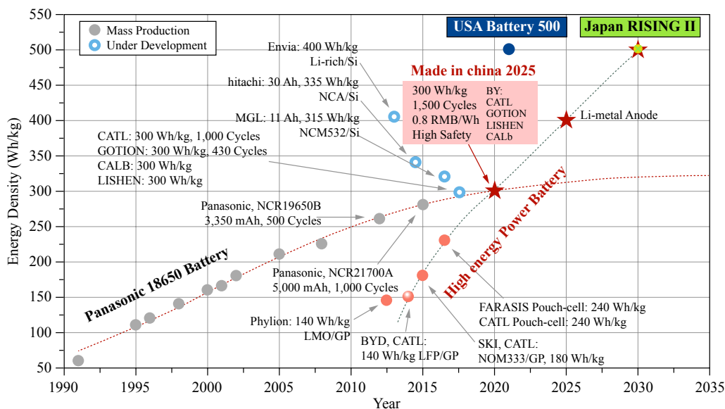
▲圖一 鋰離子電池發展之歷程 (2)
