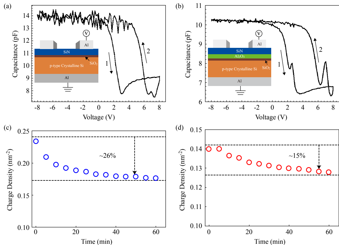
▲圖五 雙層(SiN/SiO 2 )結構之(a)電容-電壓圖；(c)電荷儲存耐久度。三層(SiN/Al 2 O 3 /SiO 2 )結構之(b)電容-電壓圖；(d)電荷儲存耐久度
